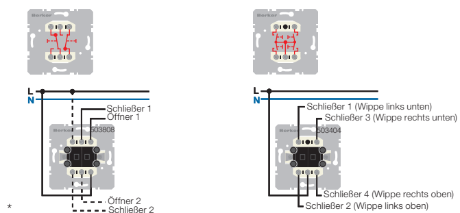
Bild 2: Serientaster, 2 Wechsler, getrennte Eingangsklemmen [Best.-Nr. 5038 08] / Gruppen-Serientaster, 4 Schließer, gemeinsame Eingangsklemme [Best.-Nr. 5034 04]
