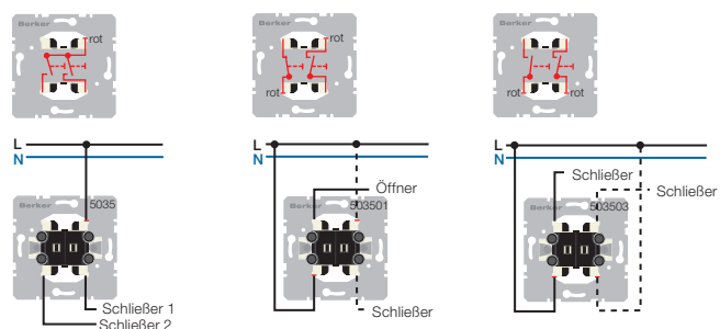
Bild 1: Serientaster, 2 Schließer, gemeinsame Eingangsklemme [Best.-Nr. 5035] / Serientaster, Öffner + Schließer, getrennte Eingangsklemmen [Best.-Nr. 5035 01] / Serientaster, 2 Schließer, getrennte Eingangsklemmen [Best.-Nr. 5035 03]
