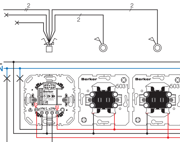
Bild 1: Universal-Tastdimmer 2fach mit Nebenstellen Taster (Schließer)
