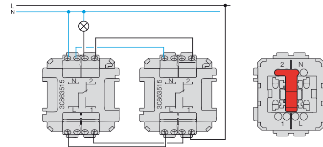
Bild 4: Beleuchtet bei EIN (Kontrollschaltung), Wechselschaltung mit 2 Kontroll-Wechselschaltern mit Linse, LED-Kontaktierung an den Klemmen 2 - 1
