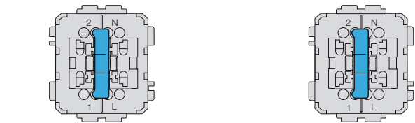
Bild 5: Beleuchtet bei AUS (Orientierungs-Beleuchtung), Kreuzschaltung mit 2 Wechselschaltern beleuchtet, mit Linse, LED-Kontaktierung an den Klemmen 2 - 1
