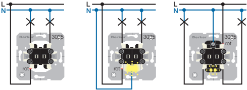
Bild 1: Serienschaltung / Serien-Kontrollschaltung: LED-Aggregat leuchtet pro Serie bei „Ein“ / Serienschaltung: Dauerbeleuchtet*
