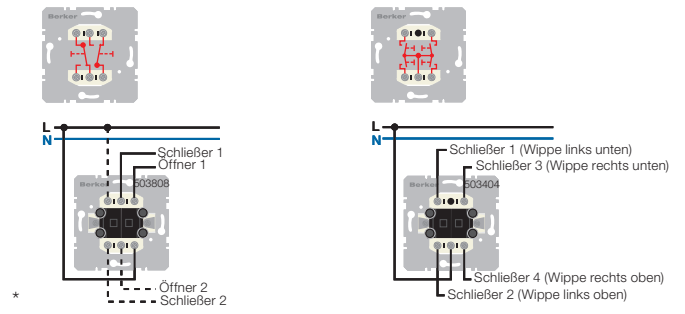
Bild 2: Serientaster, 2 Wechsler, getrennte Eingangsklemmen [Best.-Nr. 5038 08] / Gruppen-Serientaster, 4 Schließer, gemeinsame Eingangsklemme [Best.-Nr. 5034 04]
