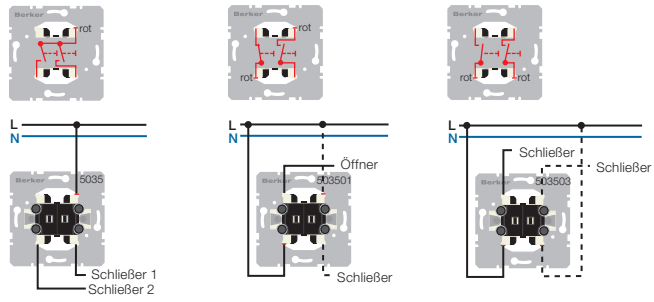
Bild 1: Serientaster, 2 Schließer, gemeinsame Eingangsklemme [Best.-Nr. 5035] / Serientaster, Öffner + Schließer, getrennte Eingangsklemmen [Best.-Nr. 5035 01] / Serientaster, 2 Schließer, getrennte Eingangsklemmen [Best.-Nr. 5035 03]
