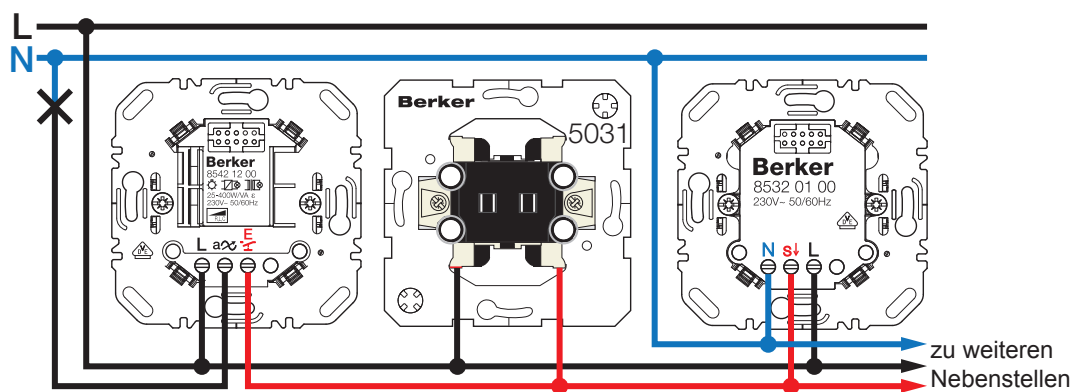
Bild 4: Tastdimmer 1fach mit Nebenstellen
