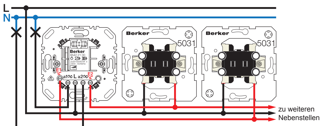
Bild 6: Tastdimmer 2fach mit Nebenstellen
