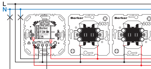
Bild 1: Universal-Tastdimmer 2fach mit Nebenstellen Taster (Schließer)
